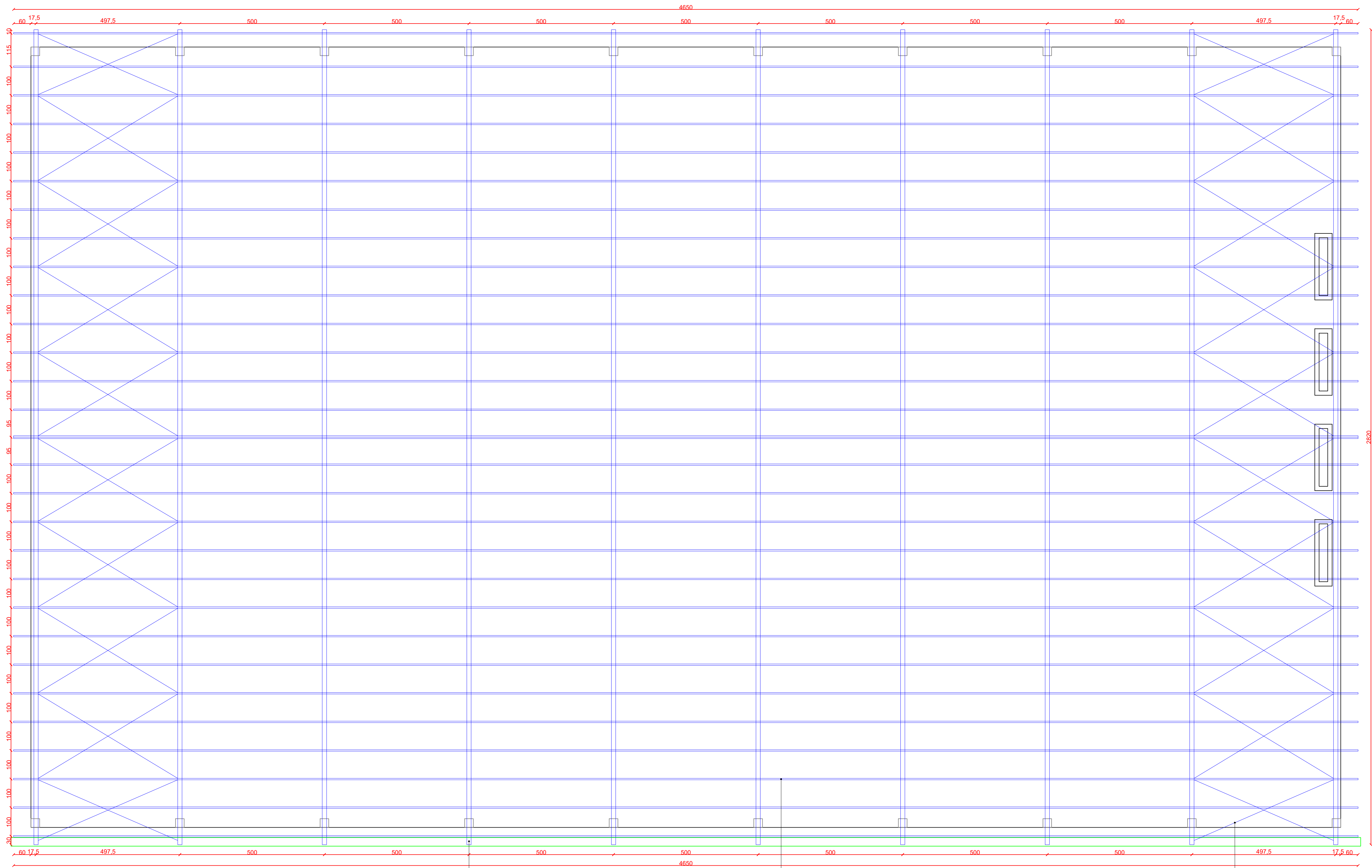
PLANTA DE LOCAÇÃO DA ESTRUTURA DE COBERTURA ESC 1/75
